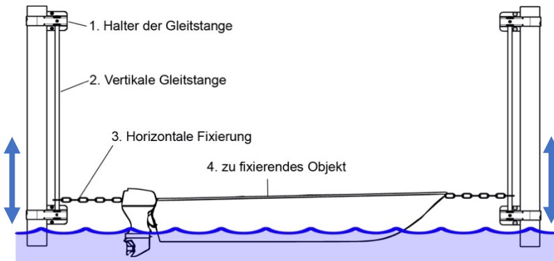
Wasserstand tief, vorne und hinten am Pfahl befestigt
