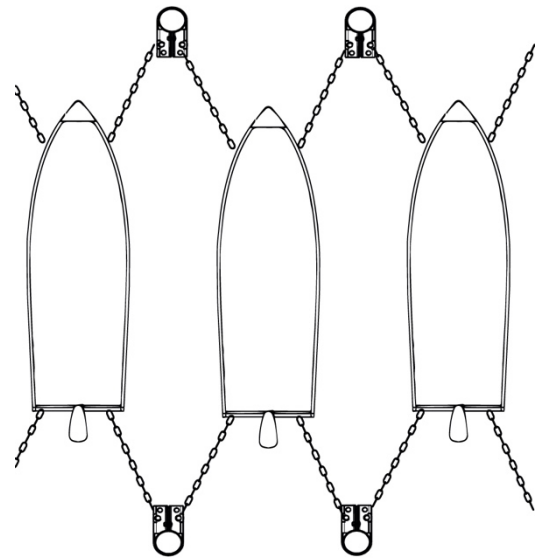
Bei jedem Wasserstand ist das Boot an den Pfählen gegen horizontale Verschiebung gesichert
