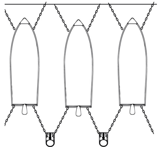
Bei jedem Wasserstand ist das Boot an den Pfählen und am Steg gegen horizontale Verschiebung gesichert
