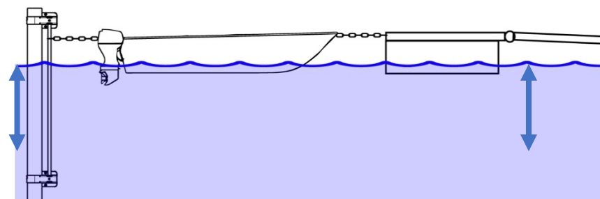
Wasserstand hoch, vorne am Schwimmsteg und hinten am Pfahl befestigt
