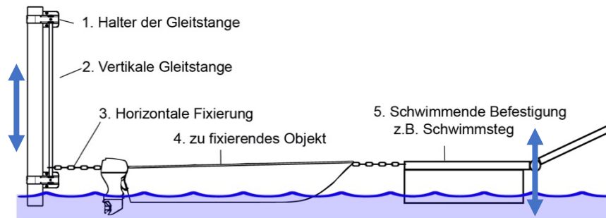
Wasserstand tief, vorne am Schwimmsteg und hinten am Pfahl befestigt
